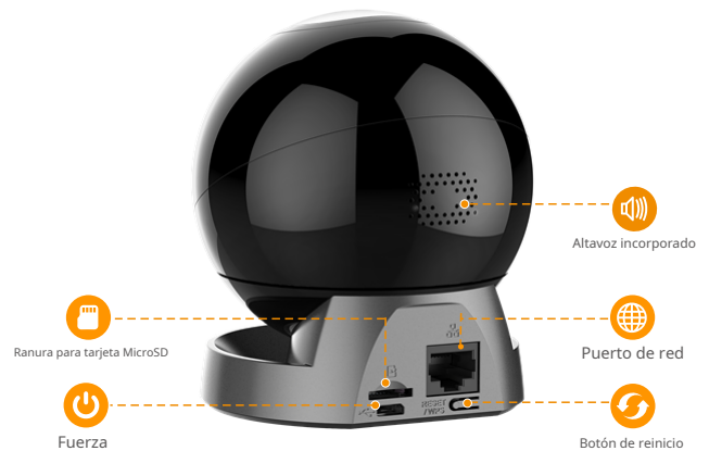
Vista trasera
