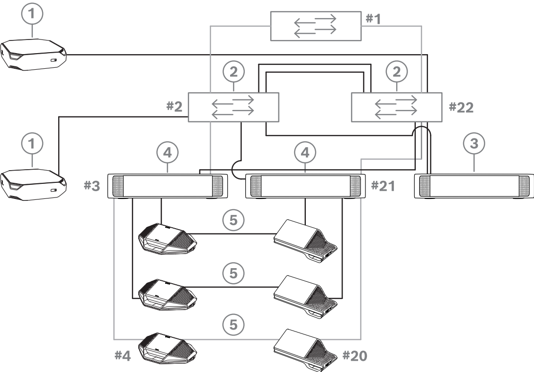
Figura 4.9: PC servidor de DICENTIS redundante con componentes y cables redundantes.
