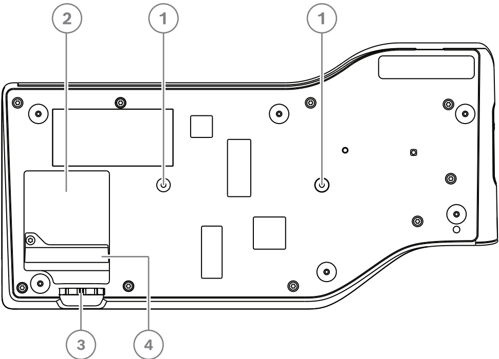
Figura 7.1: Vista inferior de los dispositivos de debate DICENTIS (DCNM-MMD / DCNM-MMD2)
