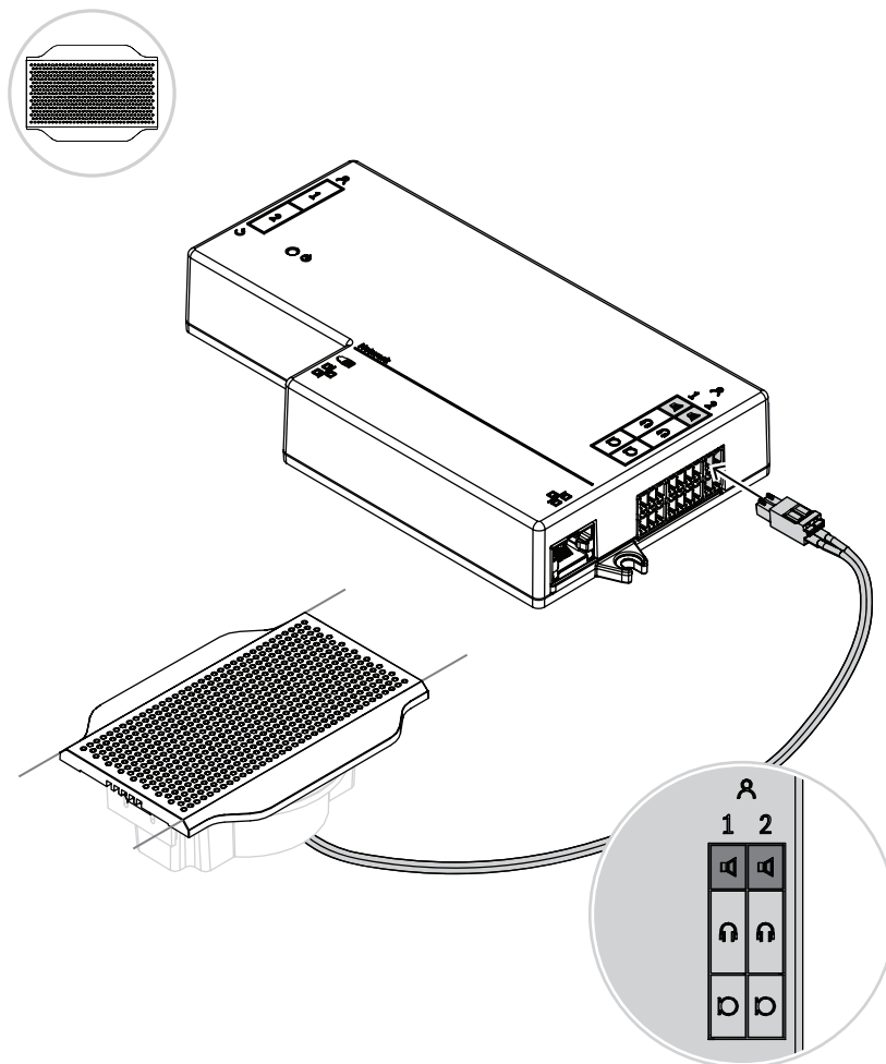
Figura 7.6: Conexión de un DCNM-FLSP al DCNM-FBD
