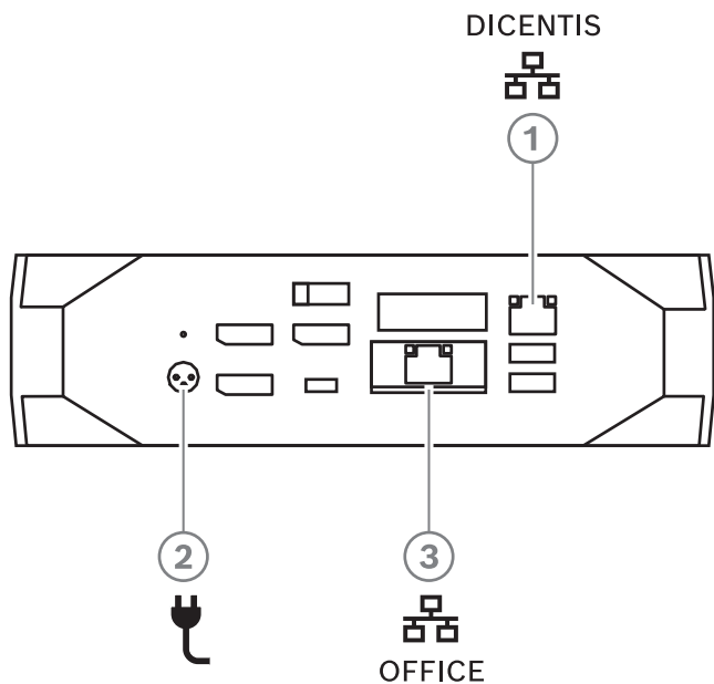
Figura 6.5: Conexiones del servidor del sistema DICENTIS
