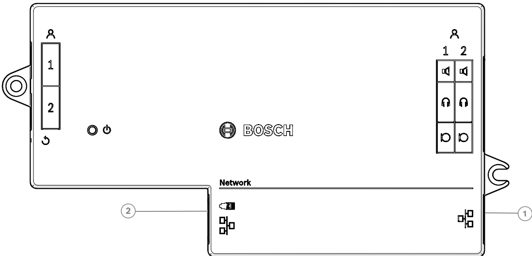
Figura 4.7: Vista superior de la unidad de base DICENTIS empotrada (DCNM-FBD)
