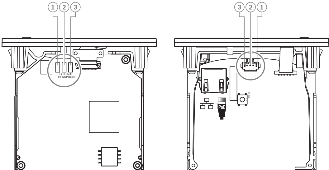
Figura 7.7: Conexión de auriculares externos
