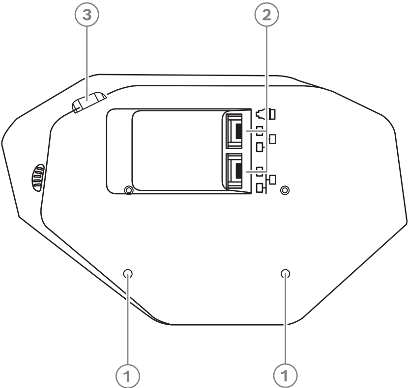
Figura 7.2: Vista inferior de los dispositivos DICENTIS (DCNM-D/DCNM-DVT/DCNM-DSL/DCNM-DE)
