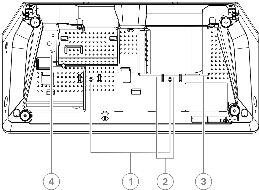
Figura 7.10: Vista inferior de DCNM-IDESK / DCNM-IDESKVID
