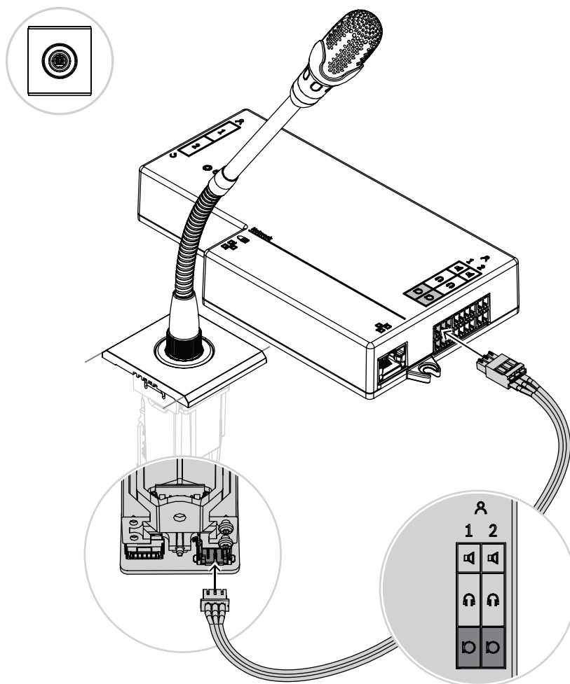
Figura 7.5: Conexión del DCNM-FMCP al DCNM-FBD
