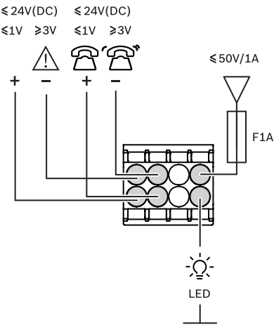
Figura 5.15: Diagrama de conexiones
