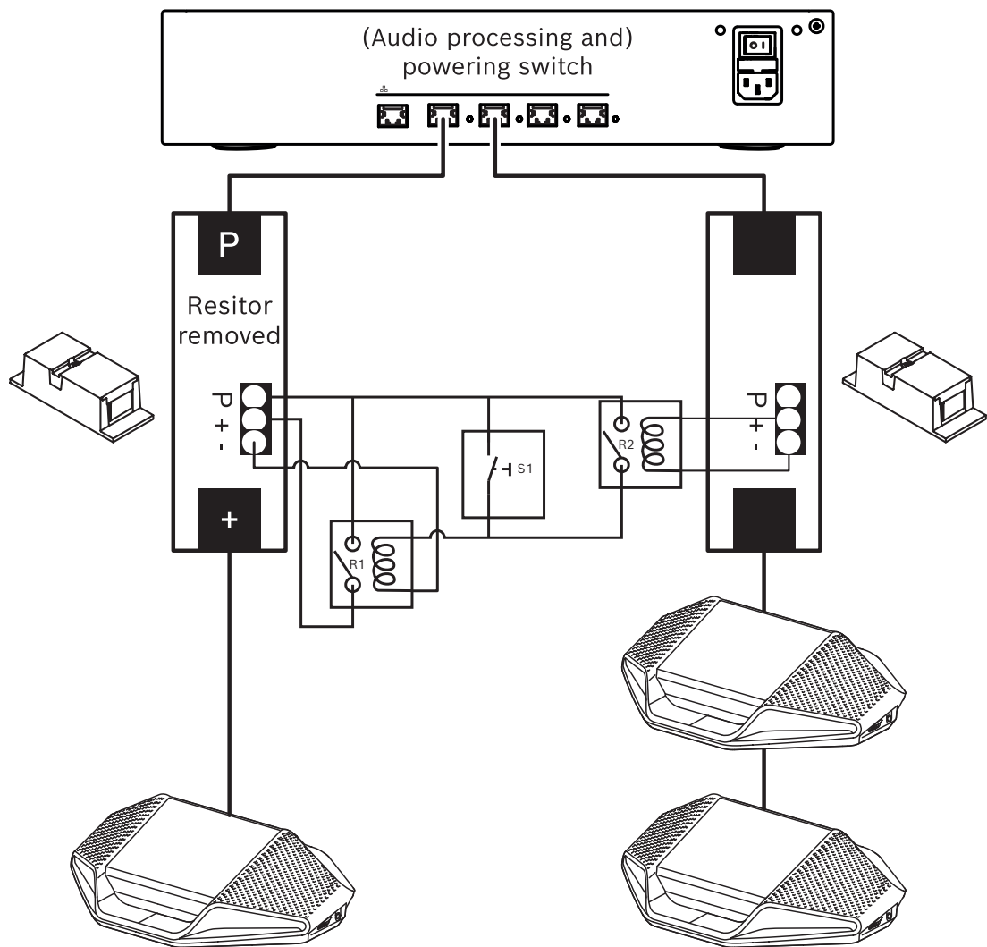
Figura 5.8: Usar acopladores de cable y un conmutador personalizado para crear un interruptor de activación
