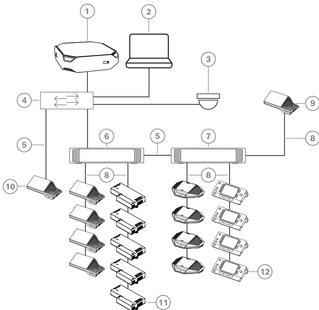
Figura 3.1: Configuración típica del sistema de conferencias DICENTIS
