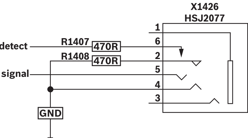
Figura 7.8: Diagrama de conector para auriculares externos
