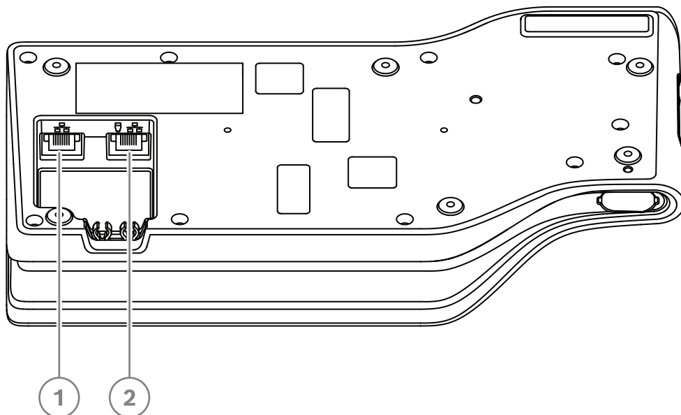
Figura 4.4: Vista inferior de los dispositivos DICENTIS (DCNM-MMD / DCNM-MMD2)
