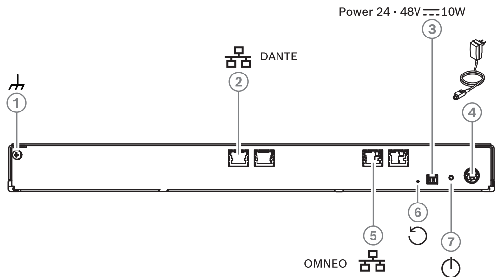
Figura 6.6: Descripción del panel posterior de OMN-DANTEGTW
