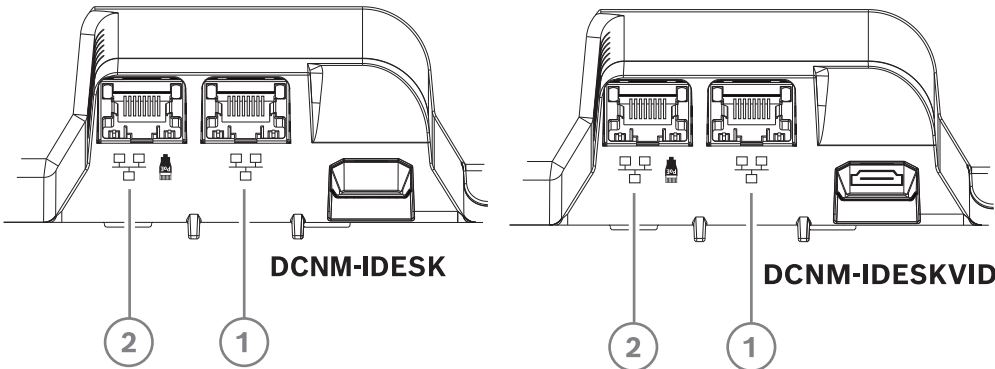
Figura 4.6: Vista inferior de los dispositivos de interpretación DICENTIS (DCNM-IDESK/DCNM-IDESKVID)
