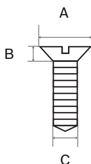
Figura 5.13: Dimensiones máximas de los tornillos
