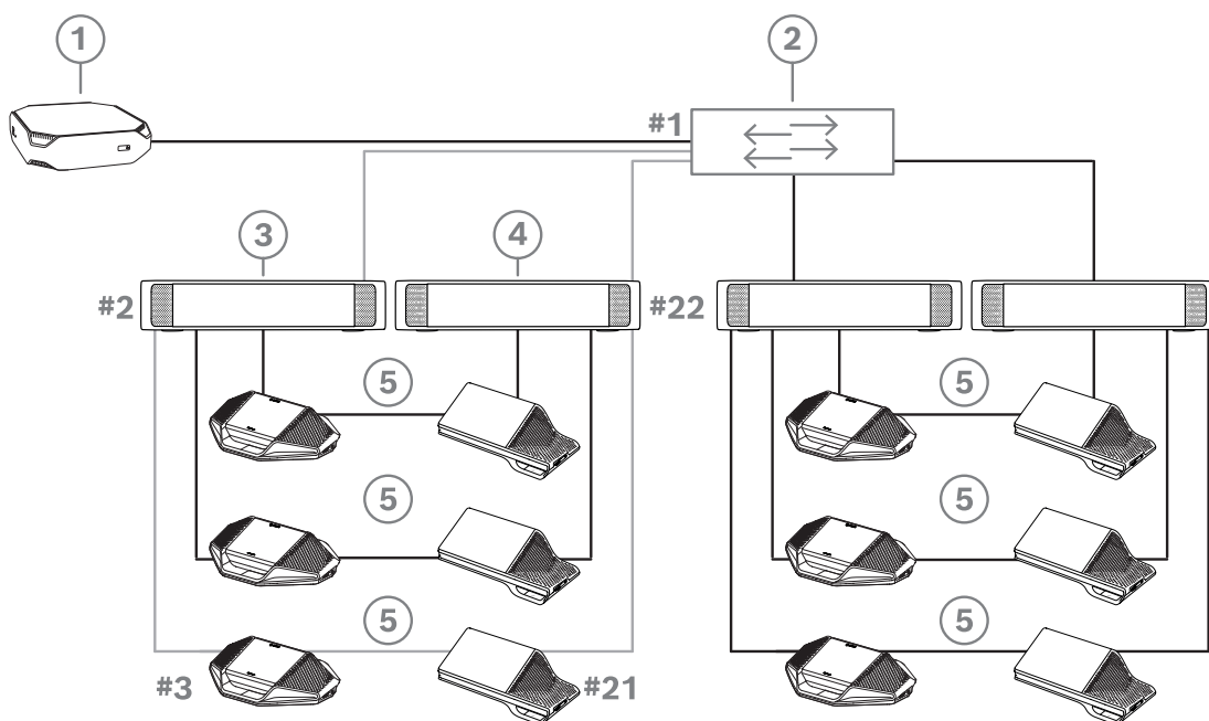
Figura 4.8: Dispositivos de debate DICENTIS con cableado redundante entre unidades de tipo DCNM-PS2/DCNM-APS2
