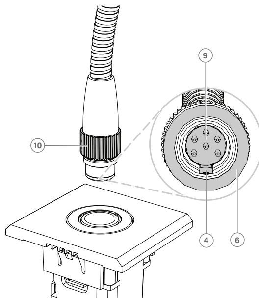
Figura 7.13: Conexión DCNM-MICSLL / DCNM-MICSL
