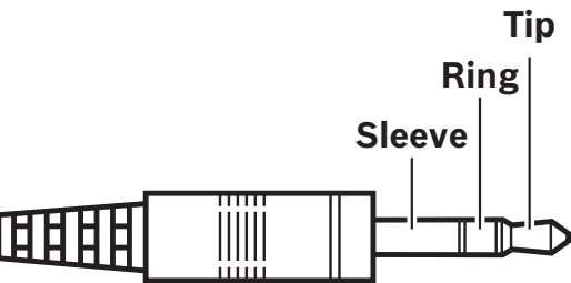
Figura 7.9: Conexión jack de auriculares
