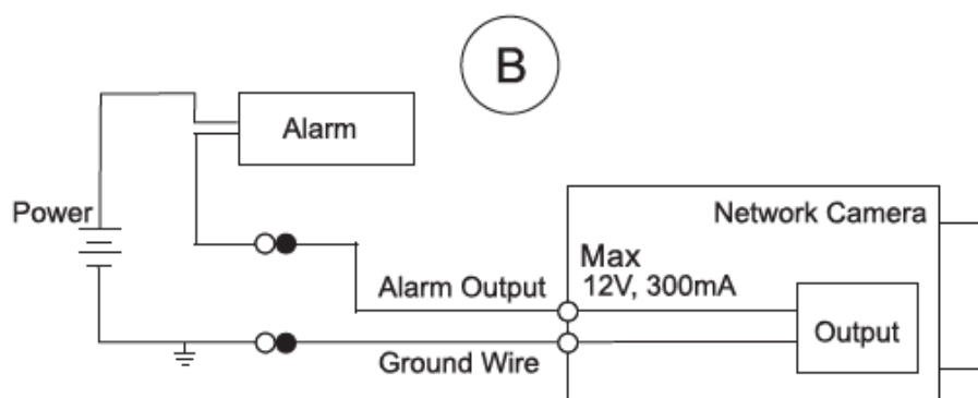
Figura 1-4 Modo B
