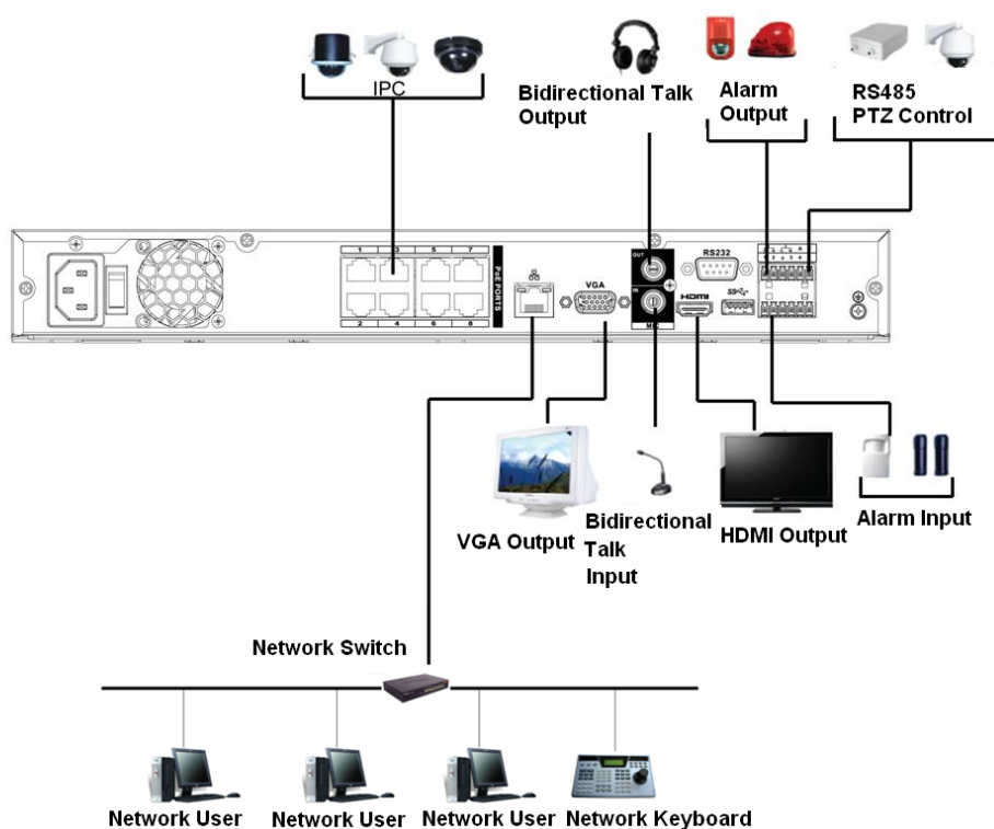
Figura 3-47 Conexión típica
