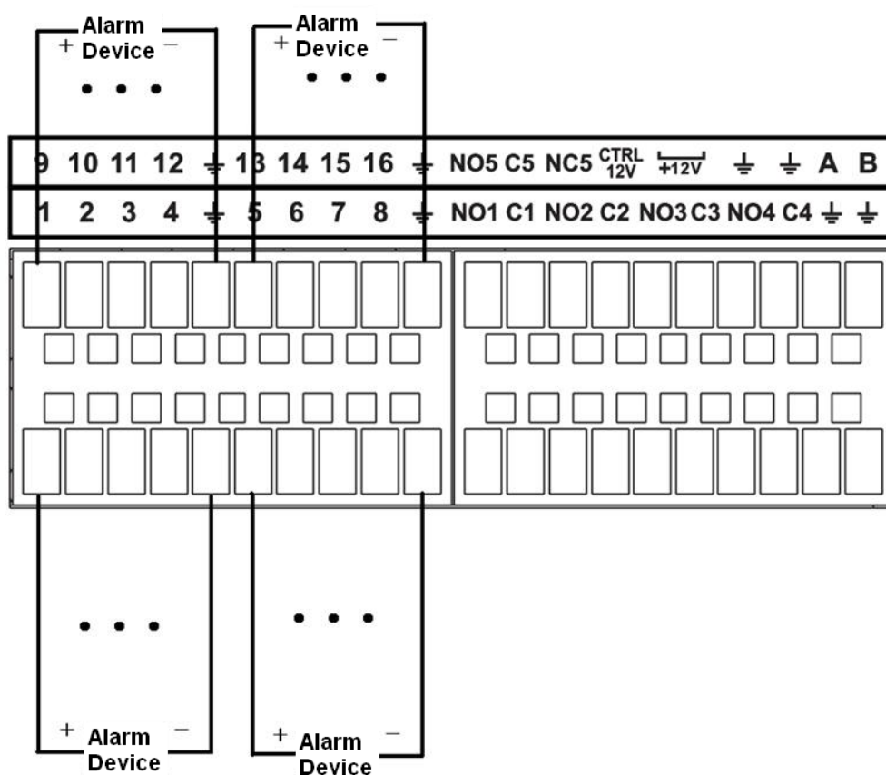
Figura 2-81 Puerto de entrada de alarma
