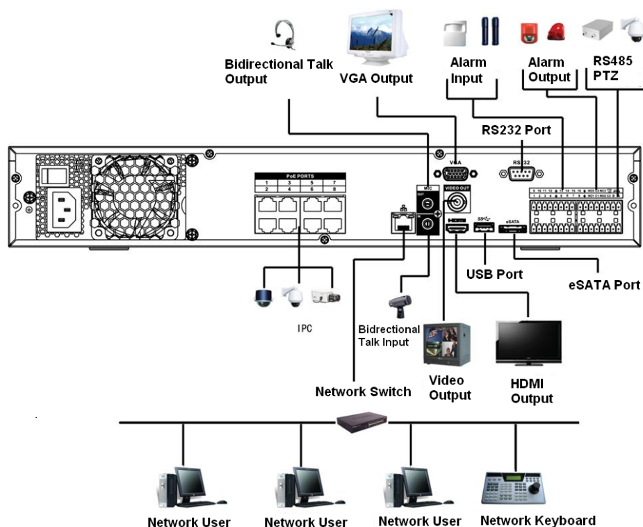
Figura 3-50 Conexión típica
