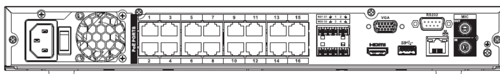
Figura 2-36 Panel trasero
