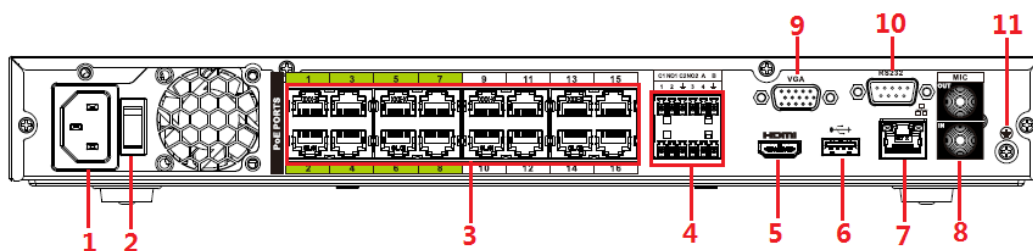
Figura 2-71 Panel trasero
