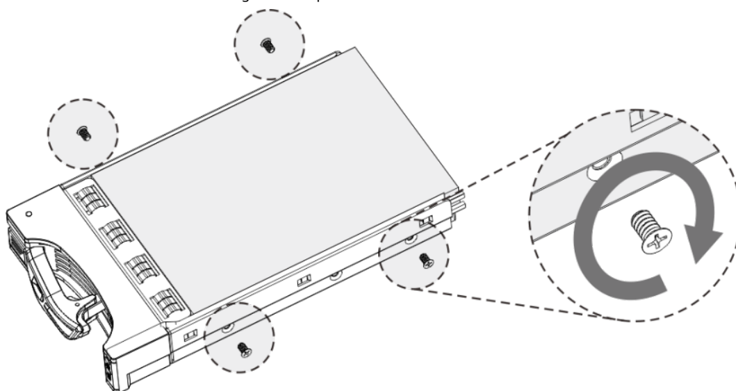
Figura 3-30 Apriete los tornillos
