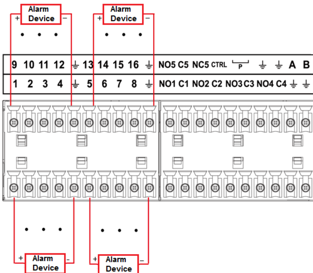
Figura 2-82 Puerto de entrada de alarma
