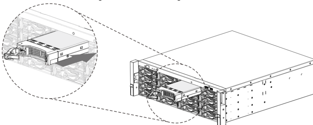
Figura 3-31 Cierre el mango
