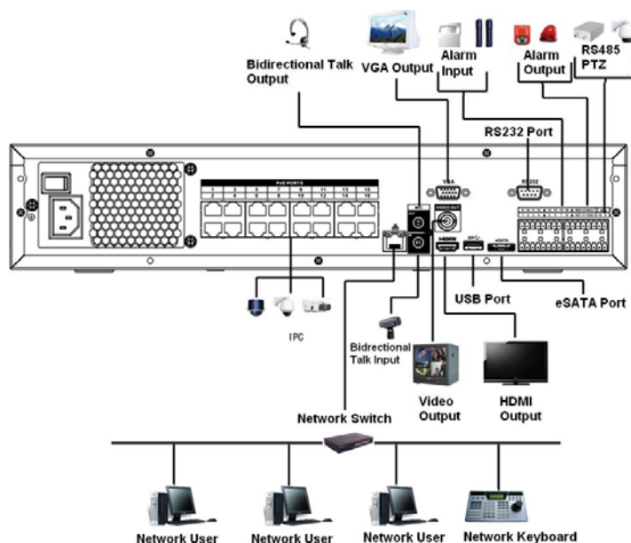
Figura 3-51 Conexión típica
