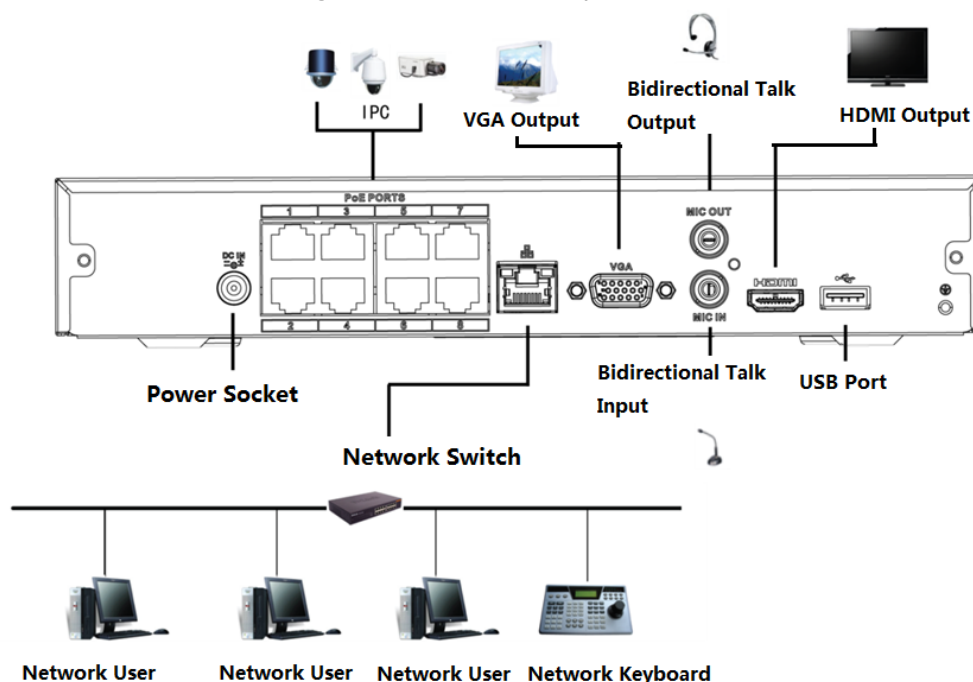
Figura 3-45 Conexión típica
