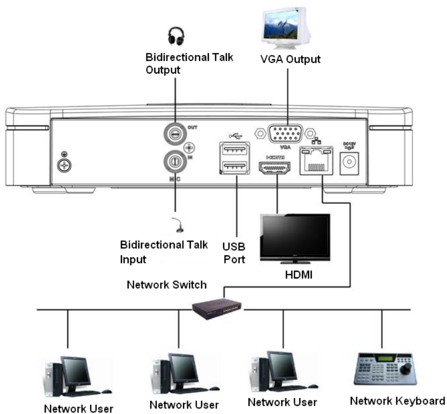
Figura 3-43 Conexión típica
