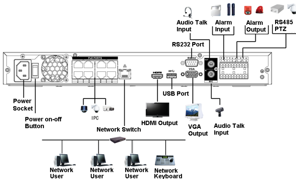
Figura 3-48 Conexión típica
