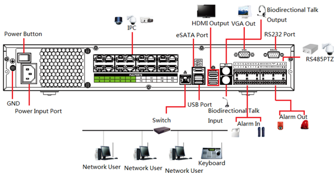
Figura 3-53 Conexión típica
