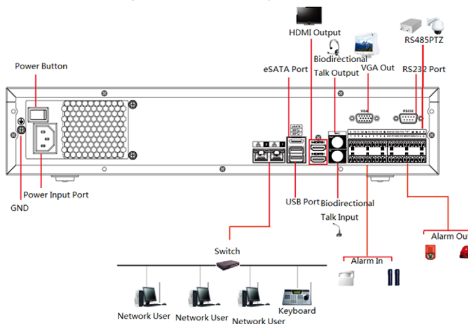
Figura 3-52 Conexión típica
