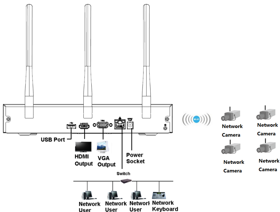
Figura 3-44 Conexión típica
