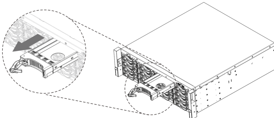
Figura 3-28 Saque la caja del disco duro
