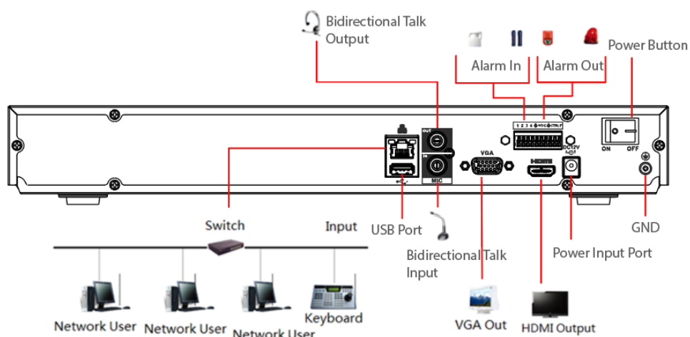
Figura 3-55 Conexión típica
