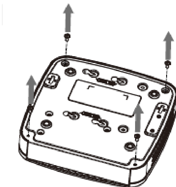
Figura 3-2 Tornillos sueltos
