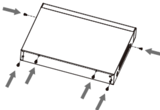
Figura 3-11 Vuelva a colocar la cubierta
