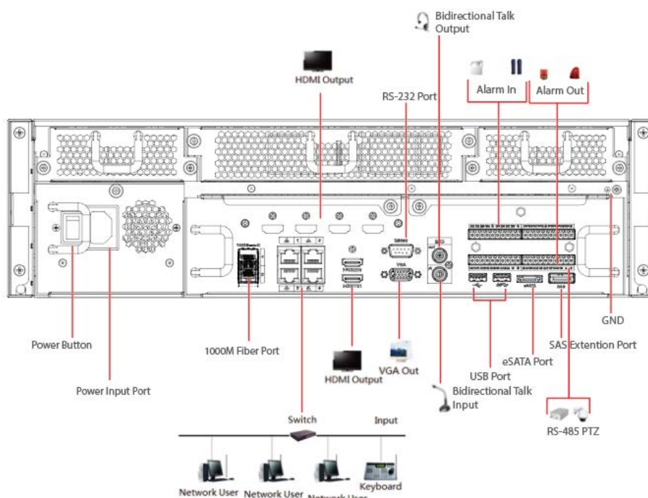
Figura 3-57 Conexión típica
