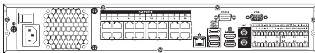
Figura 2-40 Panel trasero
