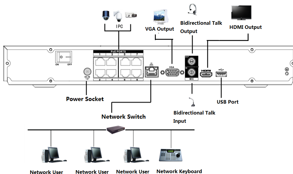
Figura 3-46 Conexión típica
