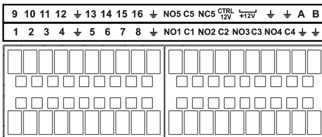
Figura 2-80 Puerto de alarma
