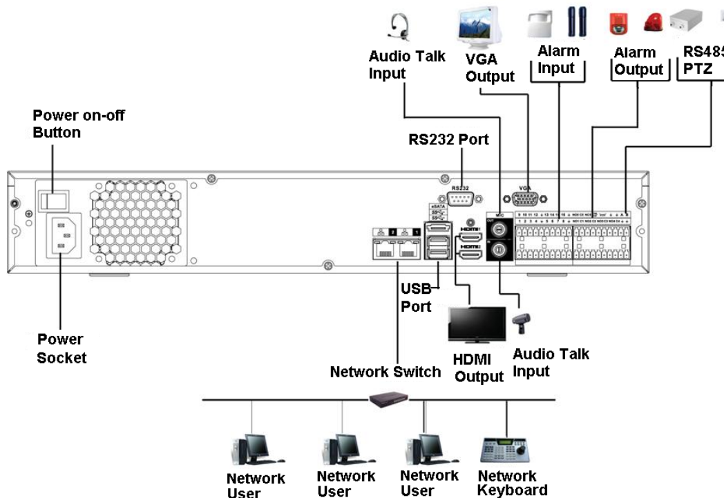
Figura 3-49 Conexión típica
