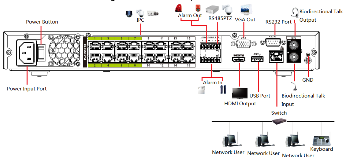
Figura 3-54 Conexión típica
