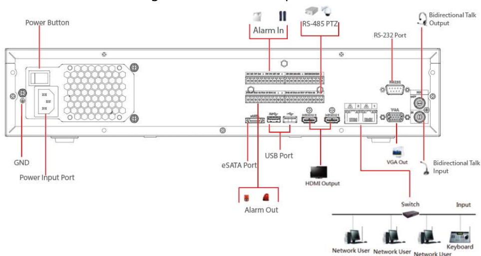
Figura 3-56 Conexión típica
