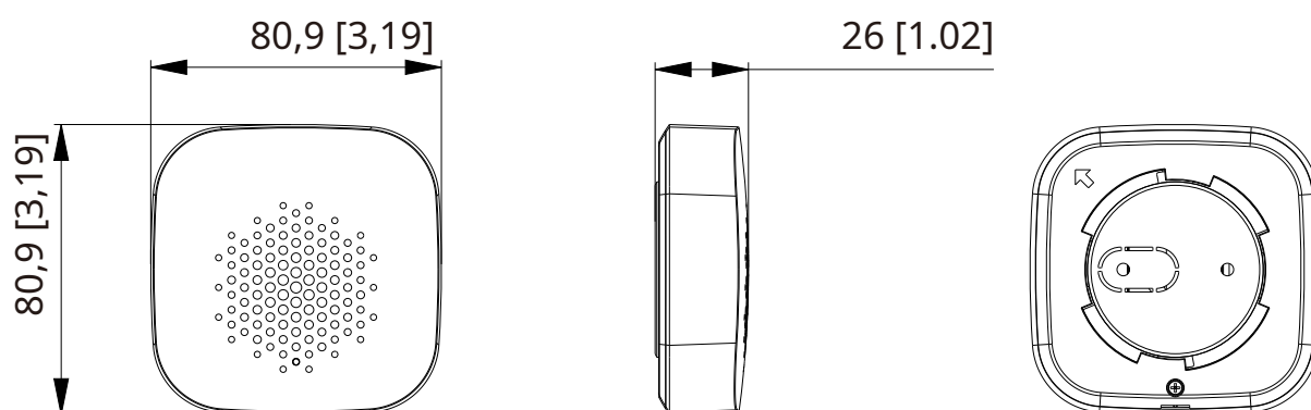
Figura 3-2 Dimensiones (mm [pulgadas])
