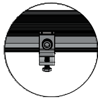
DETALLE E GROUND LUG
