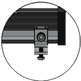
DETALLE E GROUND LUG
