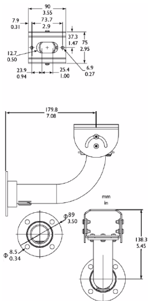
Soporte de pared corto LTC 9215/00S para uso en interiores
