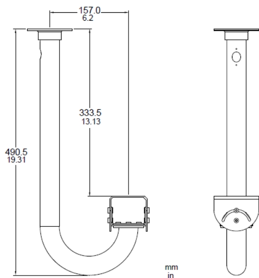
Soporte de pared corto LTC 9215/00S para uso en interiores
