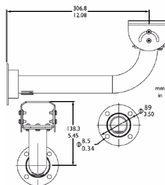
Soporte de pared LTC 9215/00 para uso en exteriores
