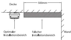
Abbildung 4-2 Installationsposition (1)
