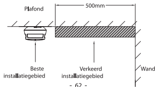
Figuur 4-2 Installatiepositie (1)
