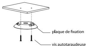
Figure 4-4 Étape d'installation (1)
