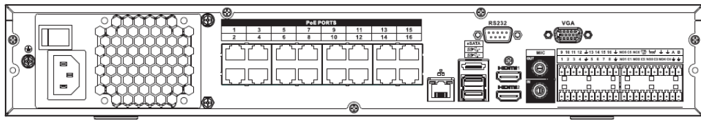
Figura 2-40 Panel trasero
