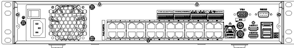
Figura 2-41 Panel trasero
