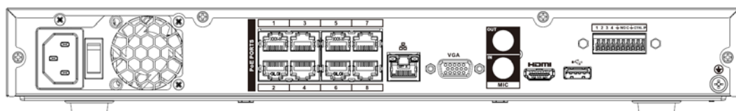
Figura 2-49 Panel trasero
