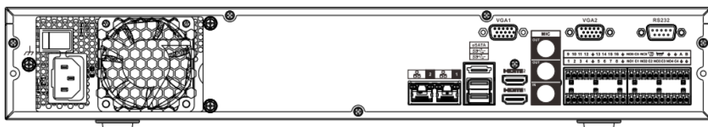
Figura 2-39 Panel trasero
