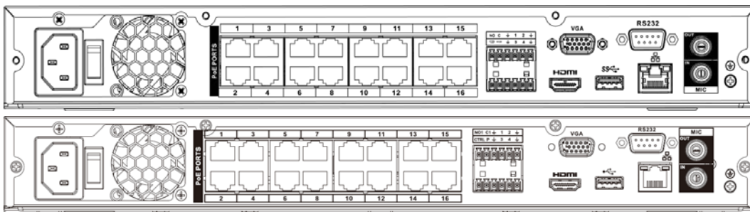
Figura 2-50 Panel trasero
