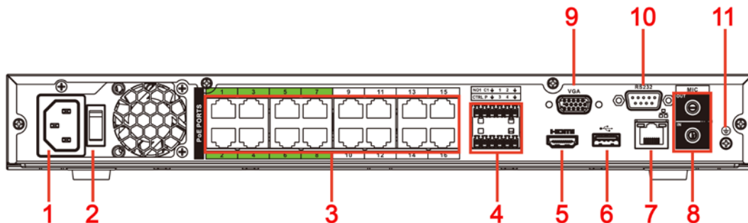
Figura 2-73 Panel trasero
