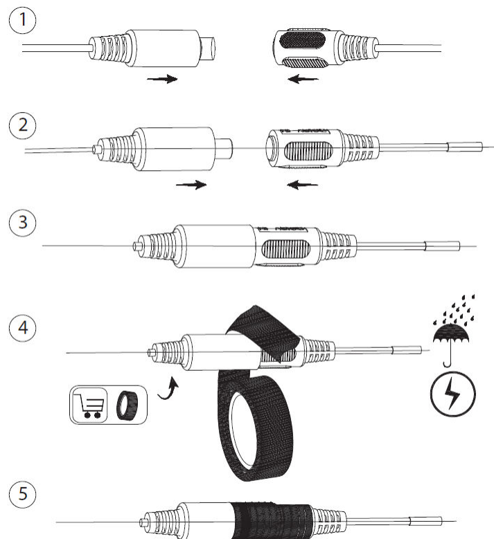
Figura 4-5 Impermeabilice el cable de alimentación
