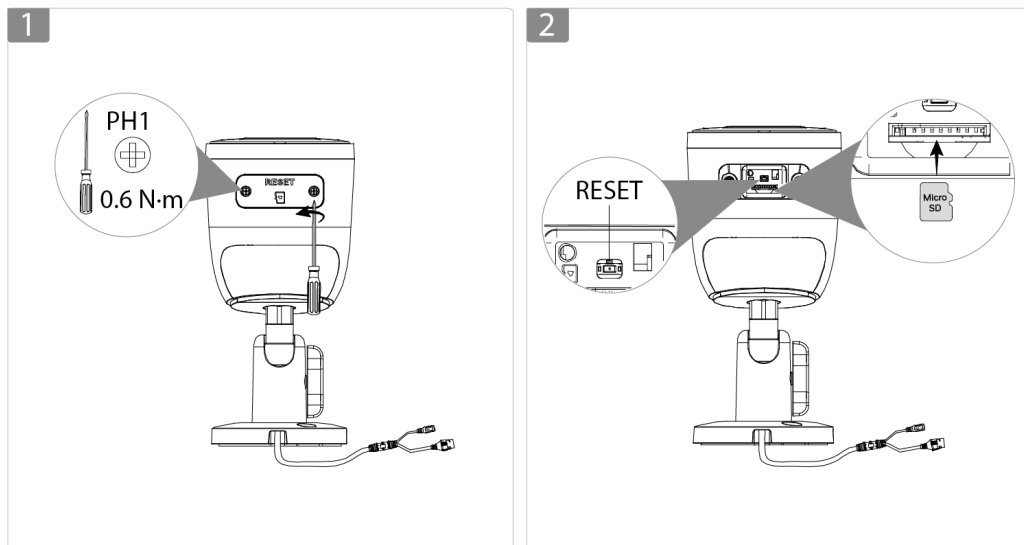
Figura 4-2 Instalar la tarjeta SD
