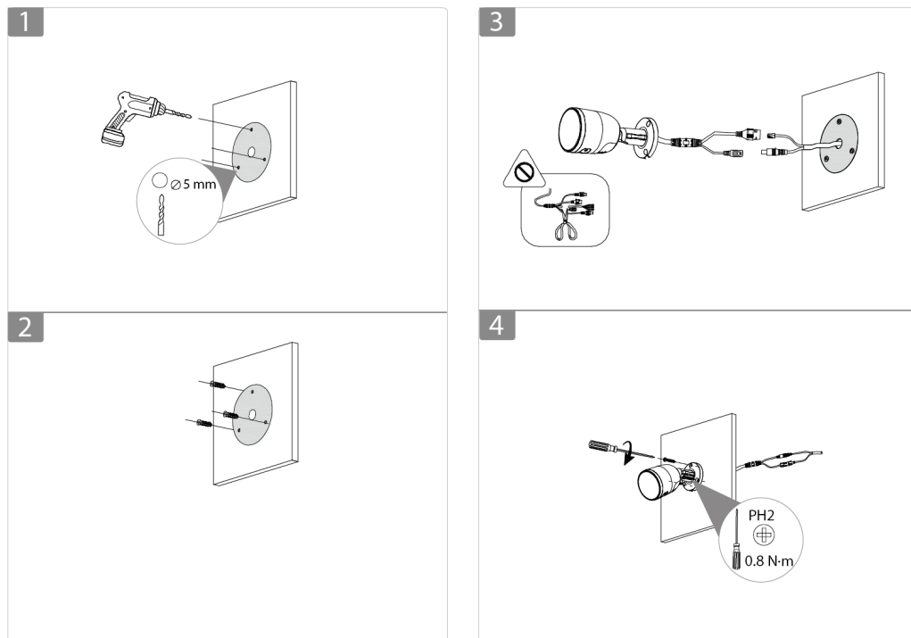
Figura 4-4 Cable que pasa por la superficie de montaje
