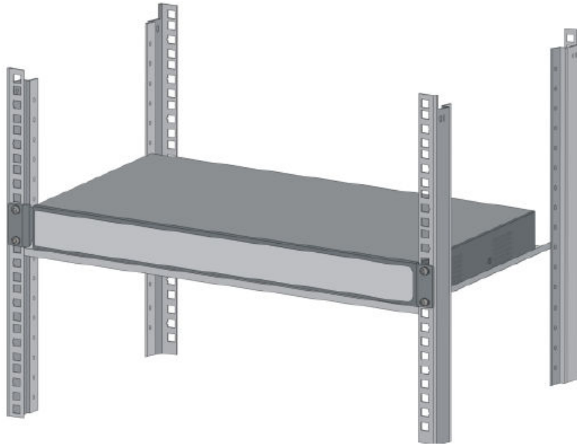
Figura 3-2 Fije el dispositivo al rack
