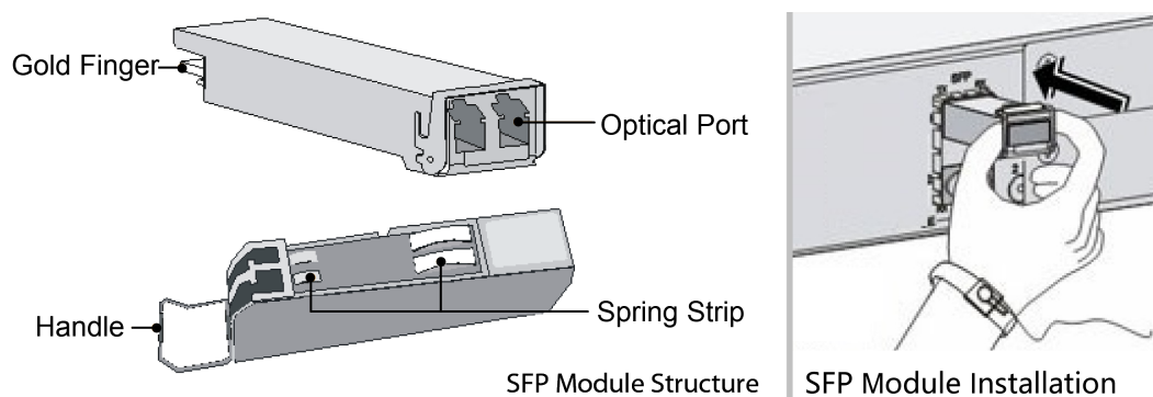
Figura 4-4 Estructura e instalación del módulo SFP
