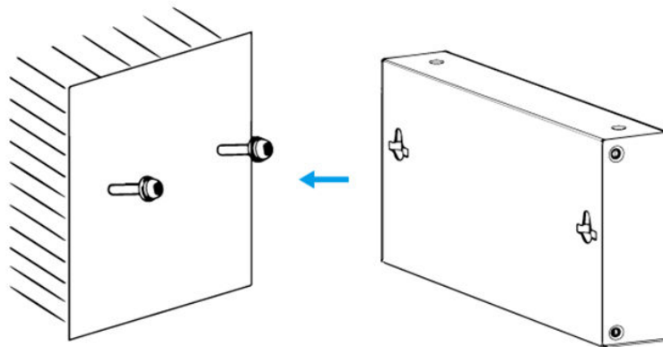
Figura 3-3 Montaje en pared
