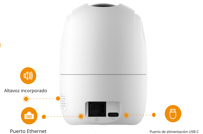
Vista posterior
