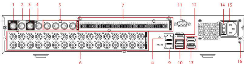
Figura 3-20 Panel trasero (2)
