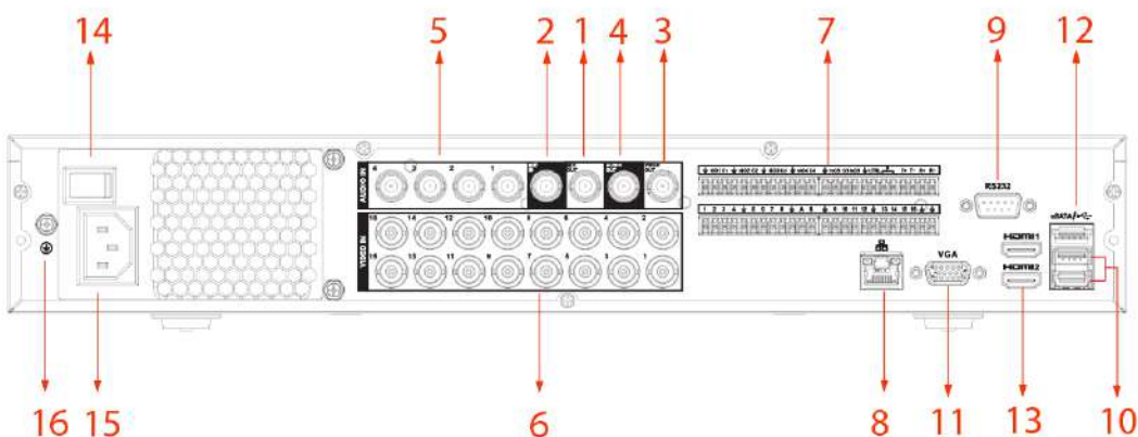
Figura 3-21 Panel trasero (3)
