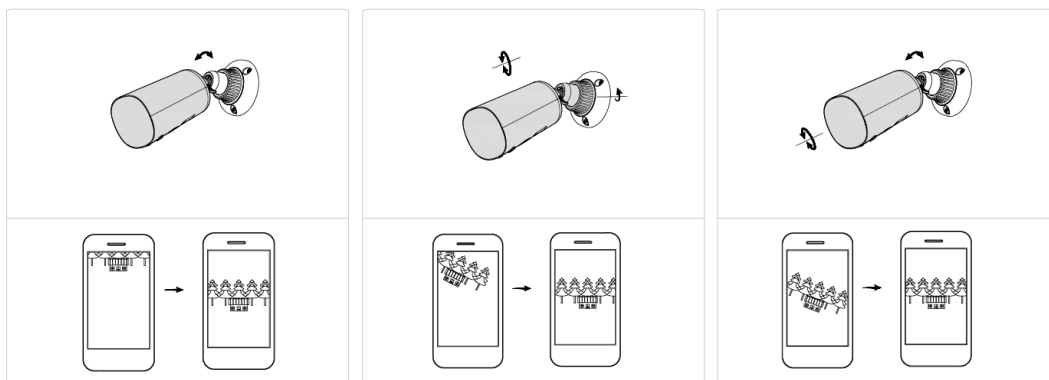
Figura 3-5 Ajuste el ángulo de la lente
