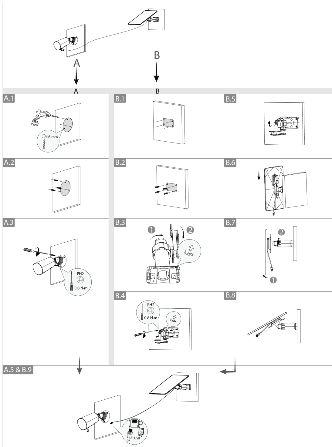
Figura 3-4 Montaje en pared
