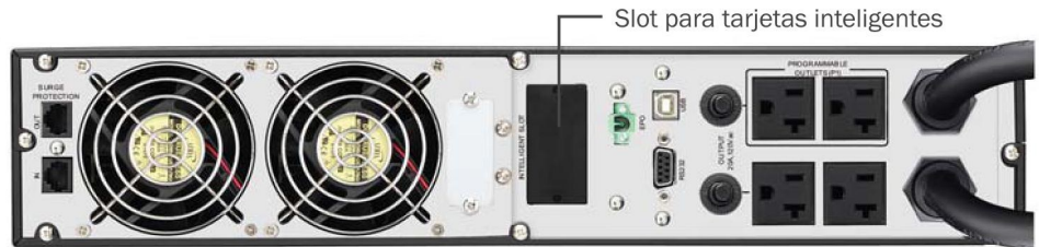
Vista trasera del equipo
