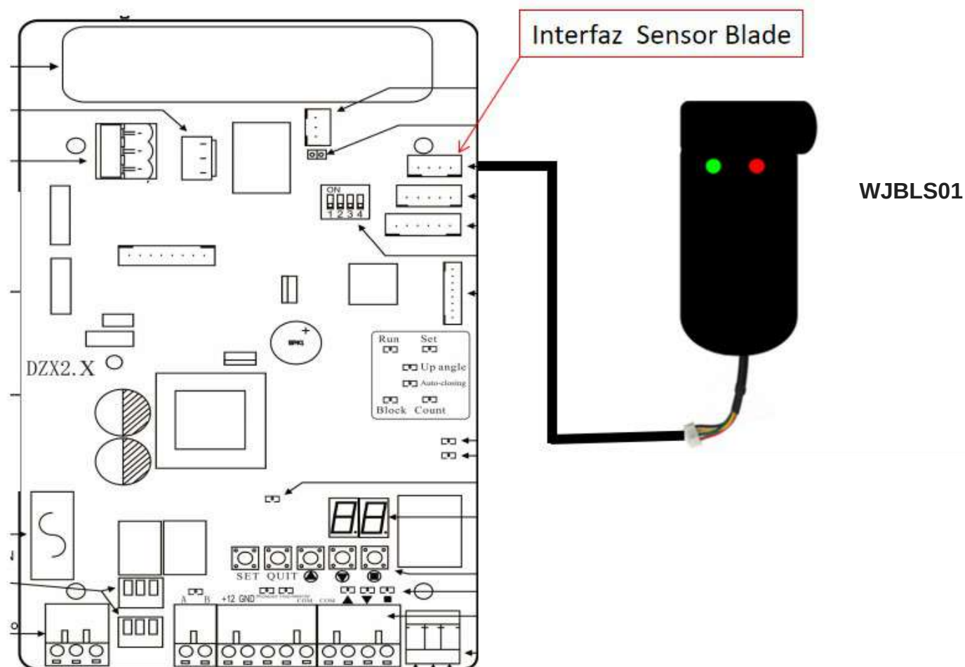
Panel de Control Barrera Vehicular Wejoin
