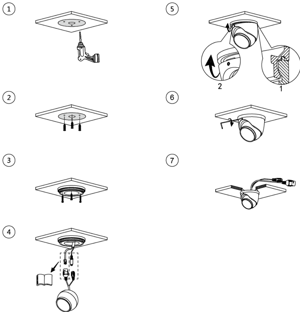
Figura 3-6 Cable que atraviesa la superficie de montaje
