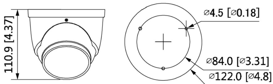
Figura 3-2 Dimensiones (Unidad: mm [pulgadas])
