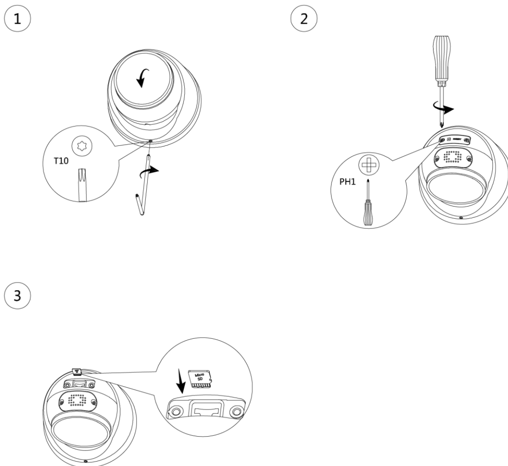
Figura 3-4 Instalación de la tarjeta SD
