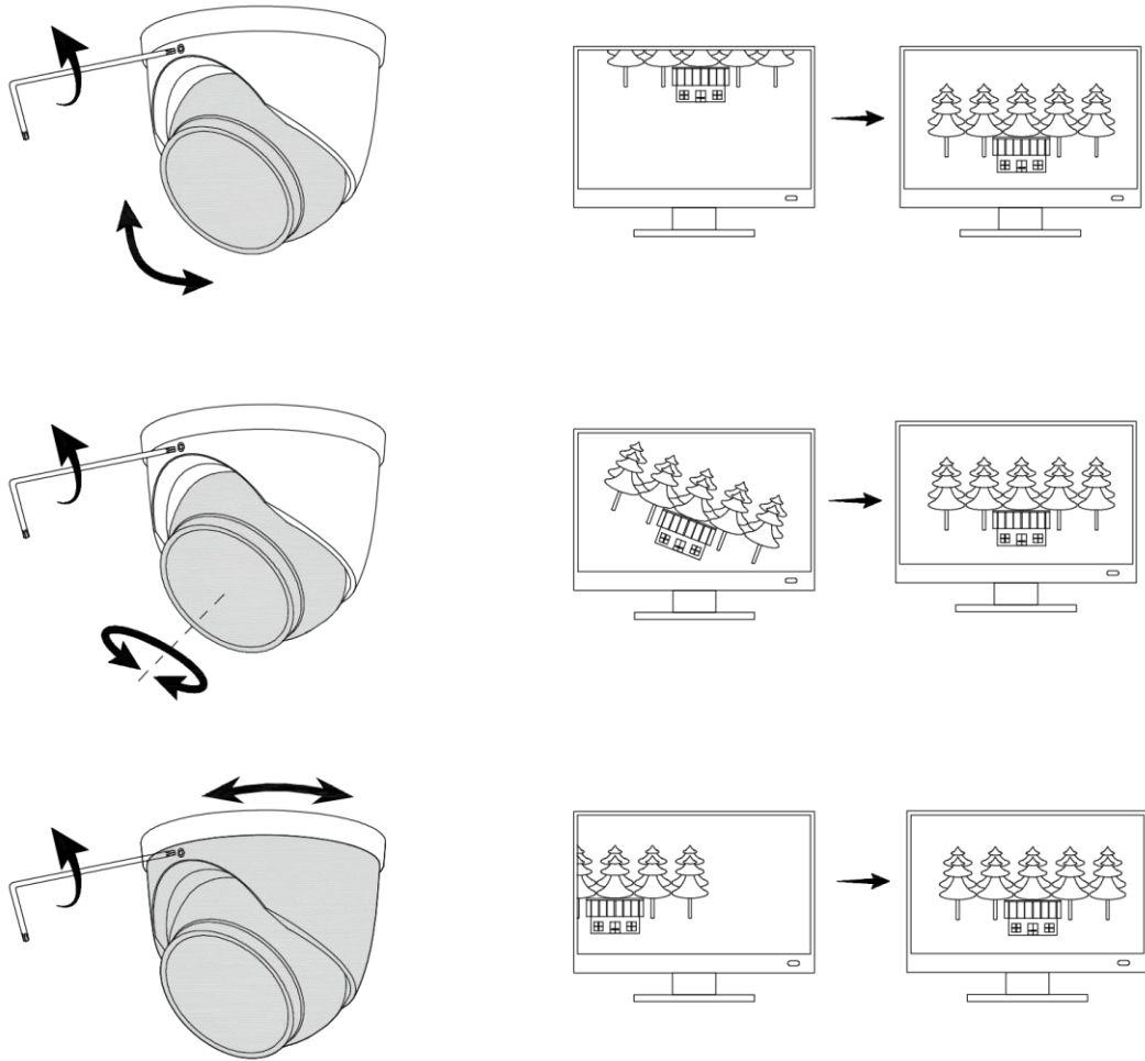
Figura 3-8 Ajuste del ángulo de la lente
