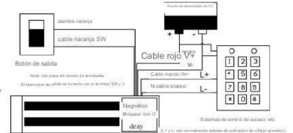
Puerta de cristal Representación de una instalación típica
