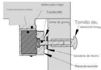
Vista en sección de la estructura de montaje para tipo colgante
