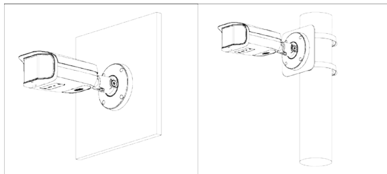
Figura 3-3 Métodos de instalación
