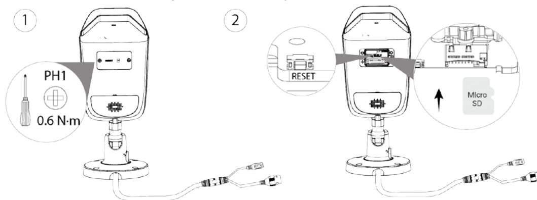
Figura 3-4 Instale la tarjeta SD
