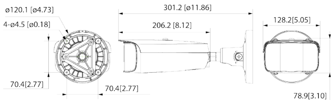
Figura 3-2 Dimensiones (mm [pulgadas])
