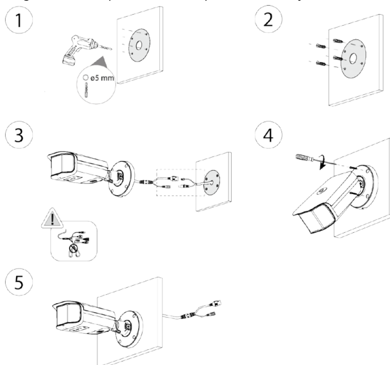
Figura 3-6 Cable que atraviesa la superficie de montaje
