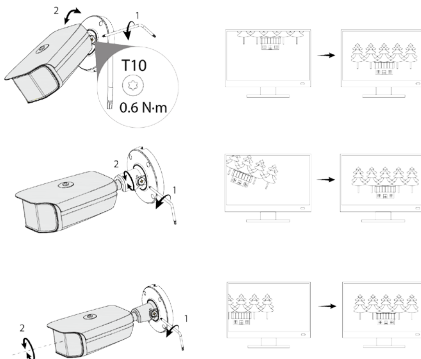
Figura 3-8 Ajustar el ángulo de la lente
