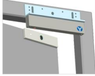
Soporte de bloqueo magnético de una puerta
